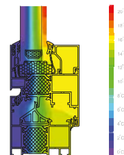
4600i 2 Multilock Izotermni Protok
